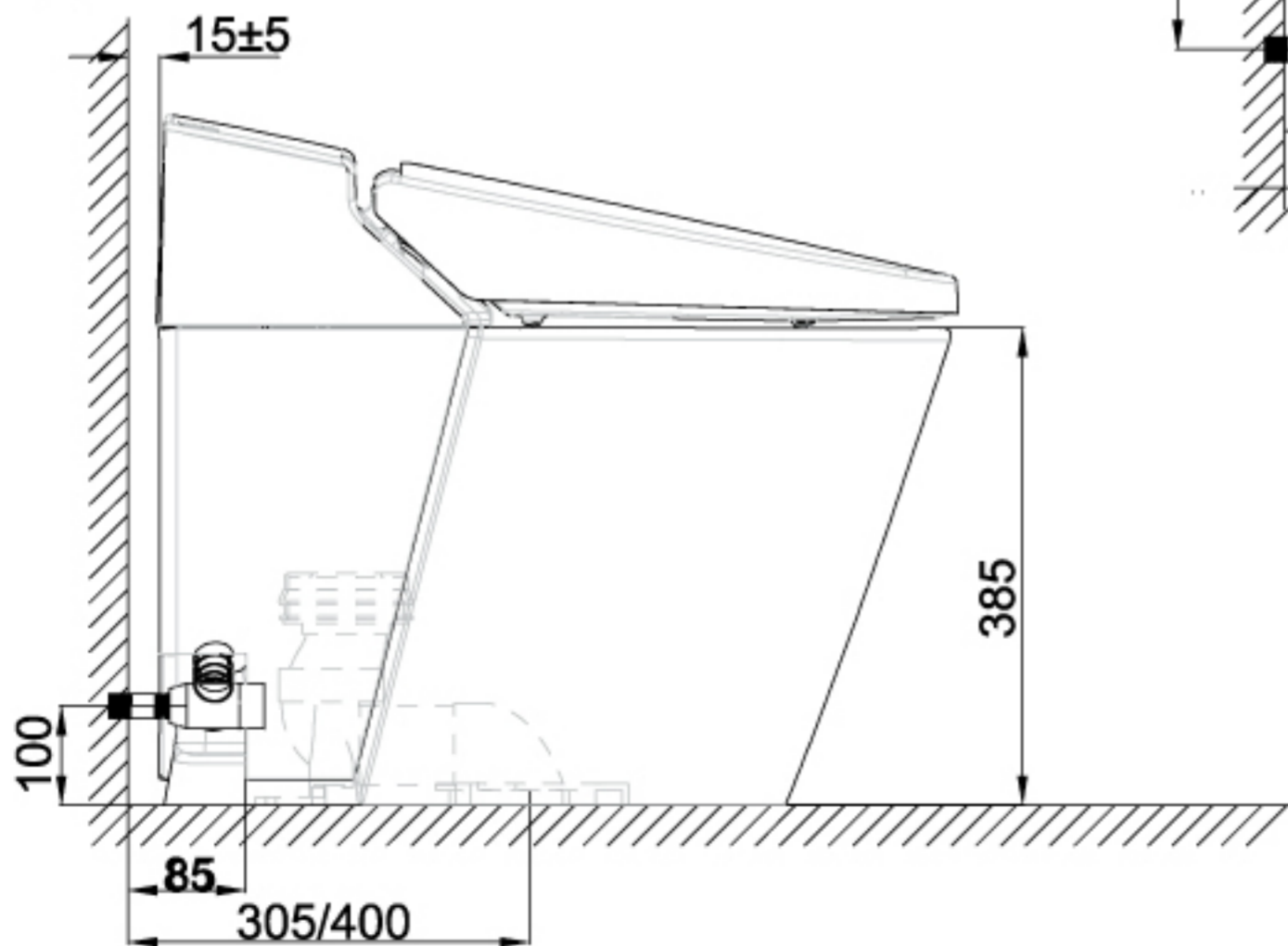
SIDE_VIEW
